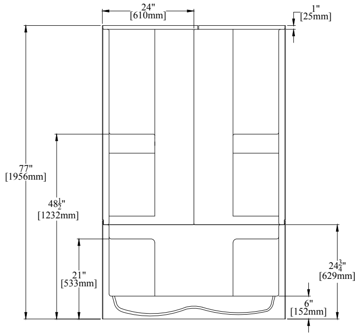
ELEVATION
